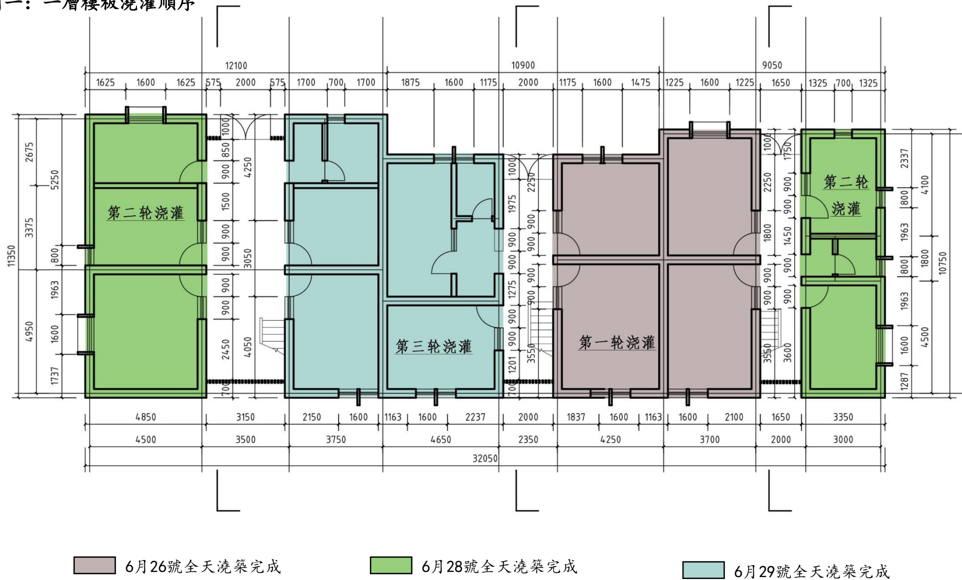
圖一：一層樓板澆灌順序
